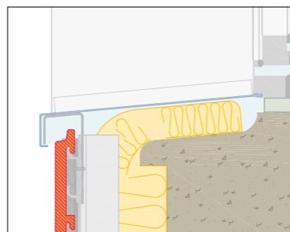
Lekdorpel
