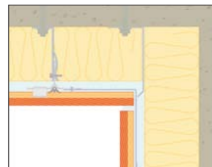
Binnenwaartse hoek
