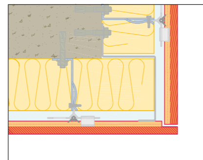
Buitenwaartse hoek
