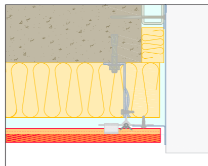
Aansluiting kozijn (metalen stijl)
